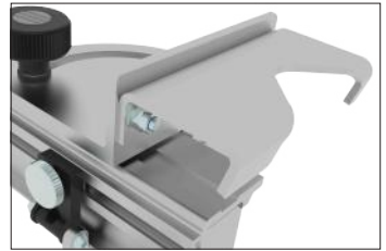
Anlehnung an Gerüststange Adossment à und barre d'échafaudage
